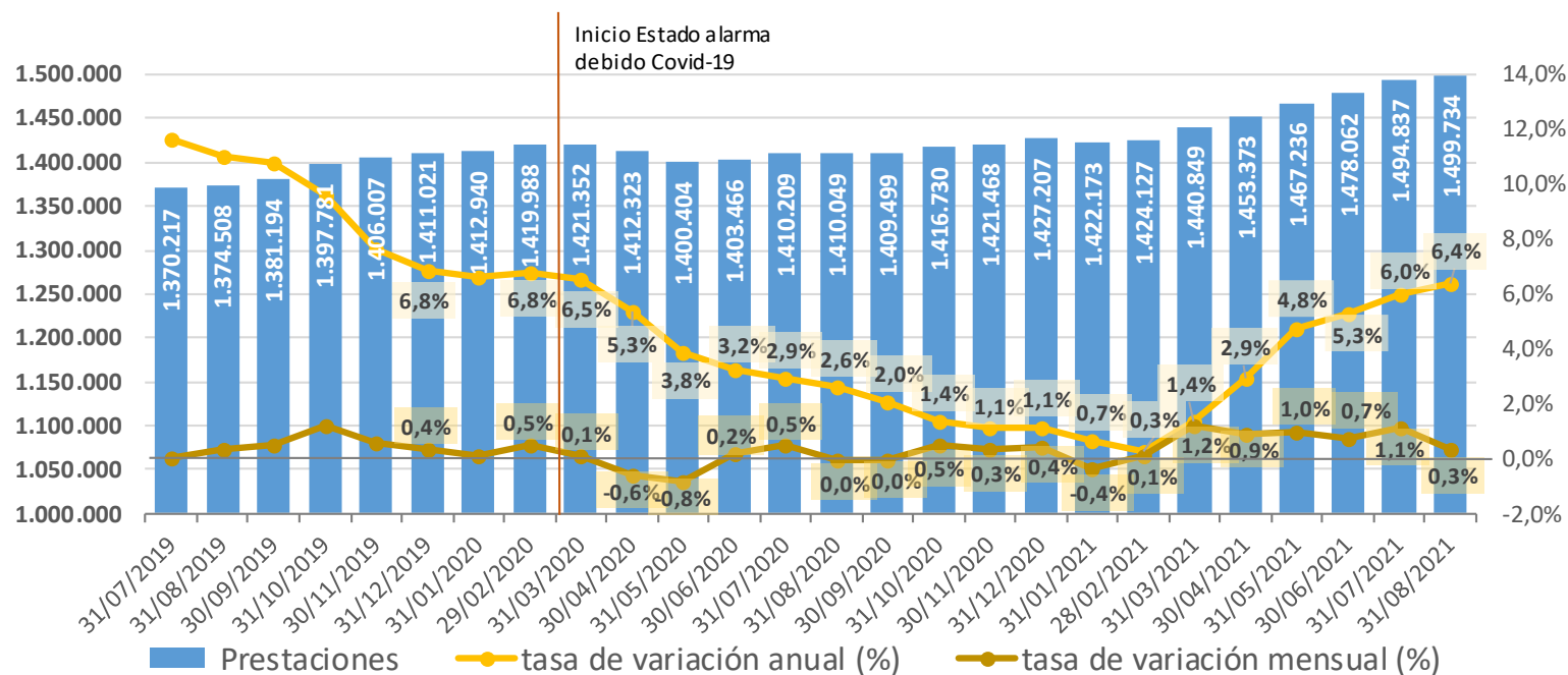
G II.- Evolución de las prestaciones
